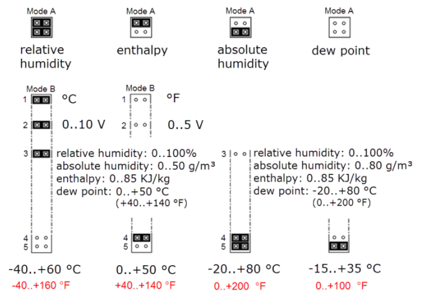
fig. (Plage de mesure et réglage offset, réglage par défaut: -20 °C..+80 °C | 0 K)
