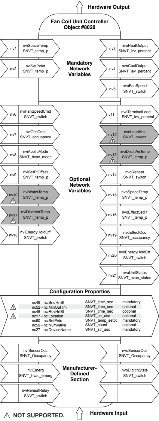
Fig. 12. LONMARK object details
